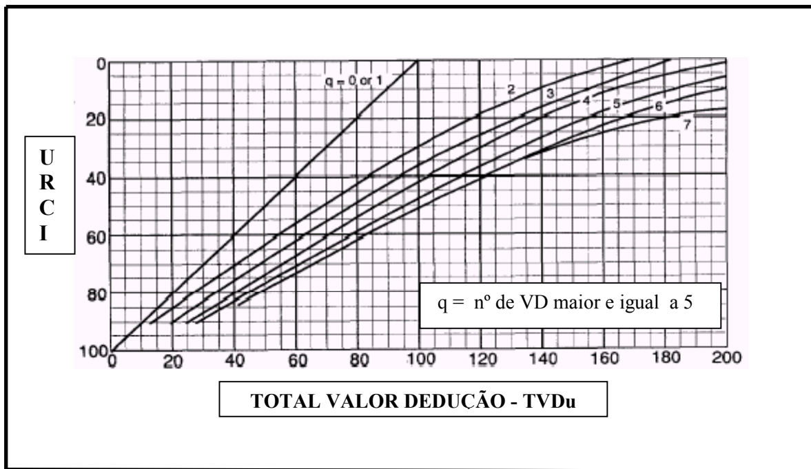
Figura B.8. Nomograma para determinação do URCI
