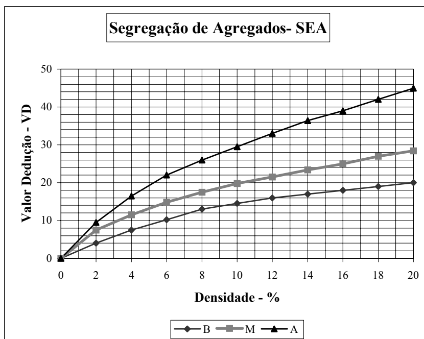
Figura B.7. Nomograma de curvas de valor-dedução – VDu: SEA - Segregação de agregados
