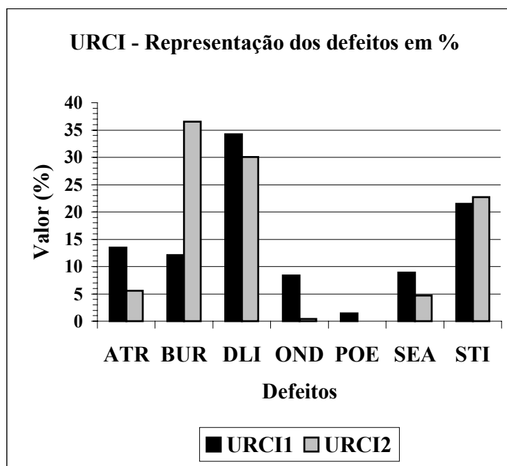
Figura 7.6. URCI - Gráfico da representação dos defeitos em %, na avaliação da estação seca – URCI1 e da chuvosa – URCI2
