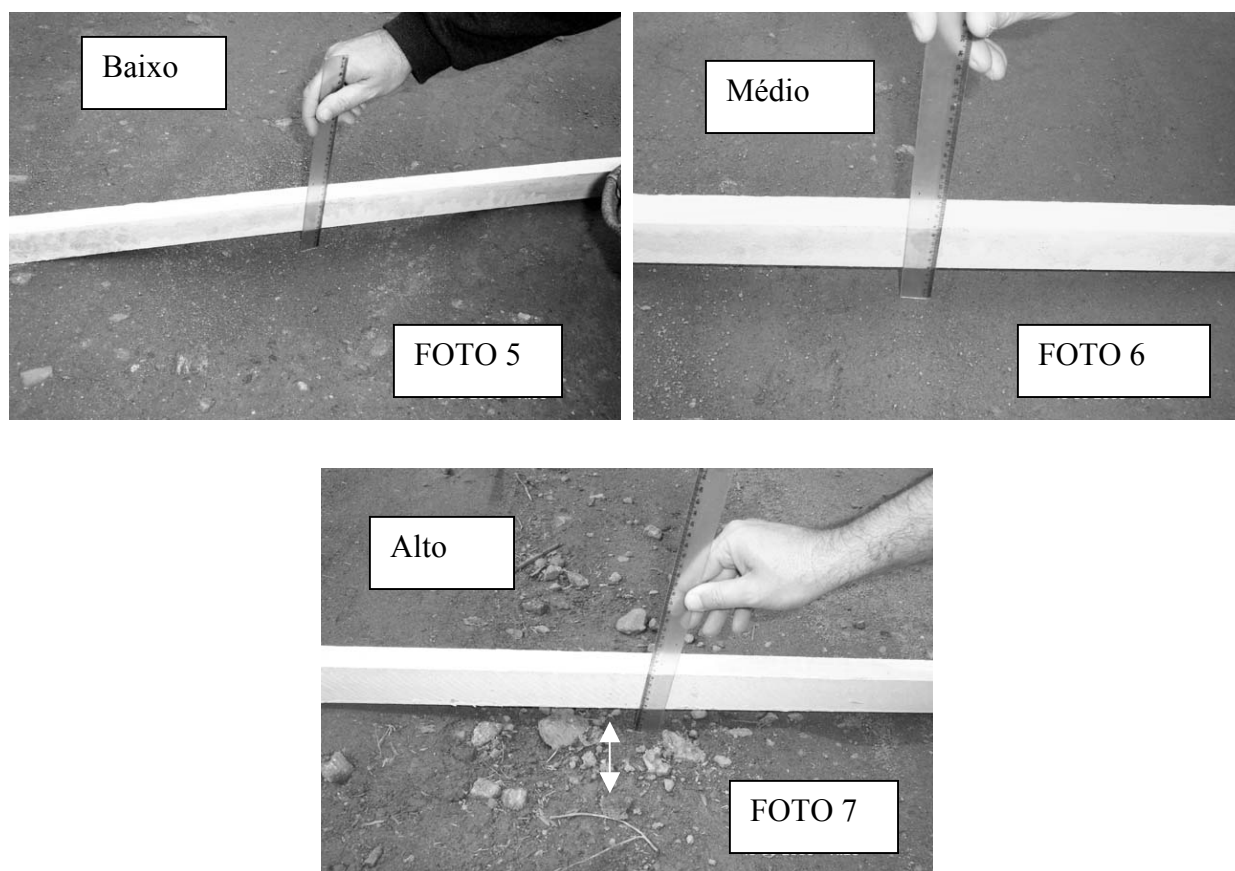
Figura 6.20. Buracos – fotografias dos níveis de severidade: fotos-5, 6,e 7
