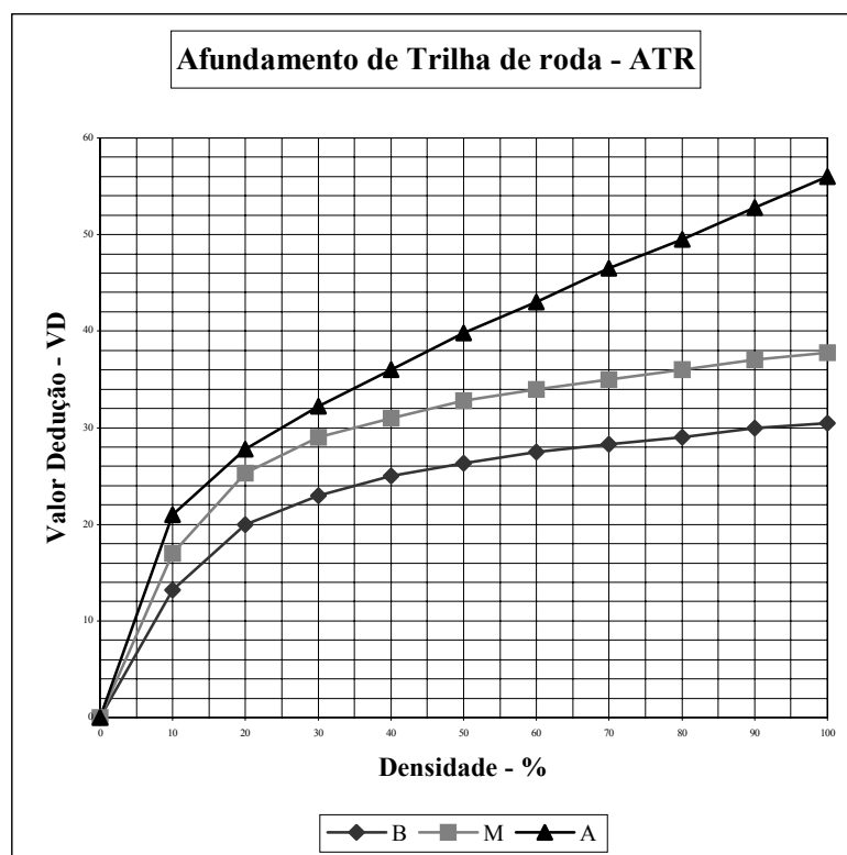
Figura B.6. Nomograma de curvas de valor-dedução – VDu: ATR – Afundamento de Trilha de Roda
