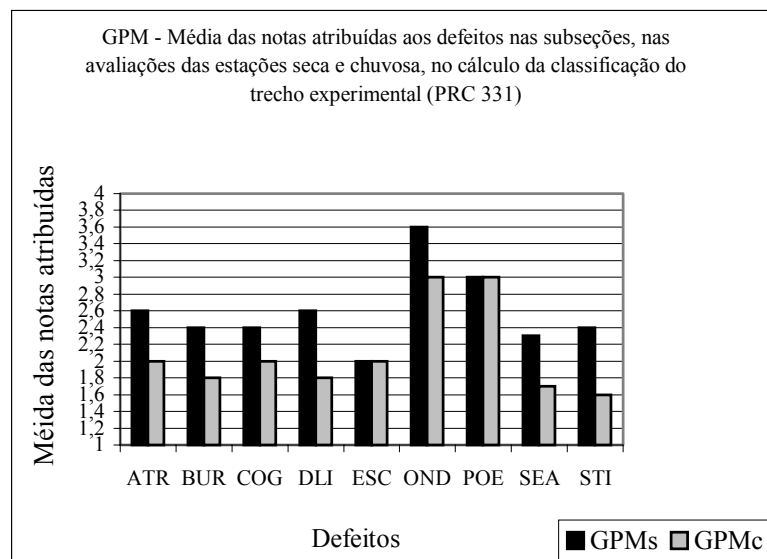
Figura 6.12. GPM - Média das notas atribuídas aos defeitos, nas avaliações das subseções, nas estações seca e chuvosa, no cálculo da classificação do trecho experimental (PRC 331)
