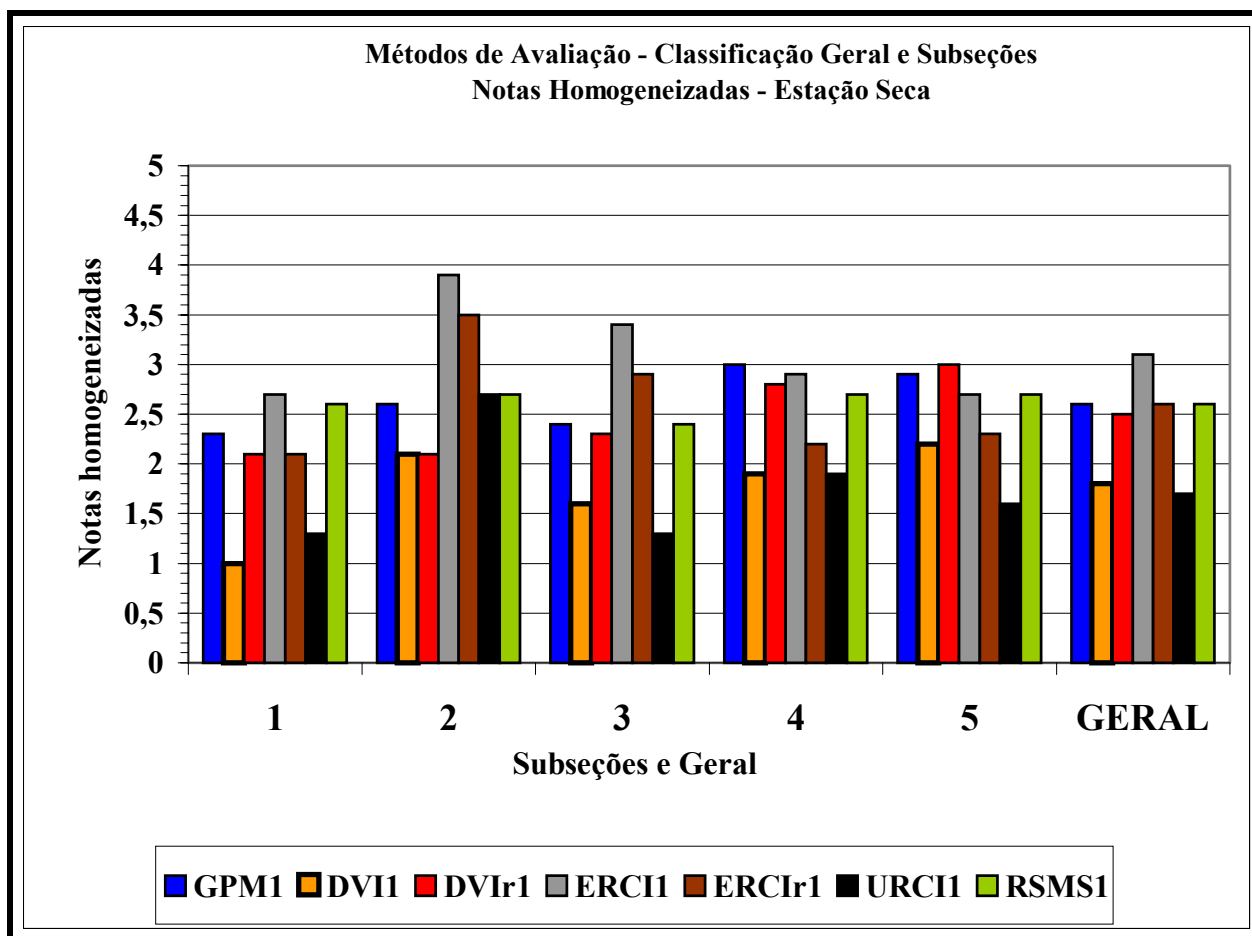
Figura 7.1. Gráfico das notas homogeneizadas das subseções e geral pelos métodos aplicados em campo na estação seca
