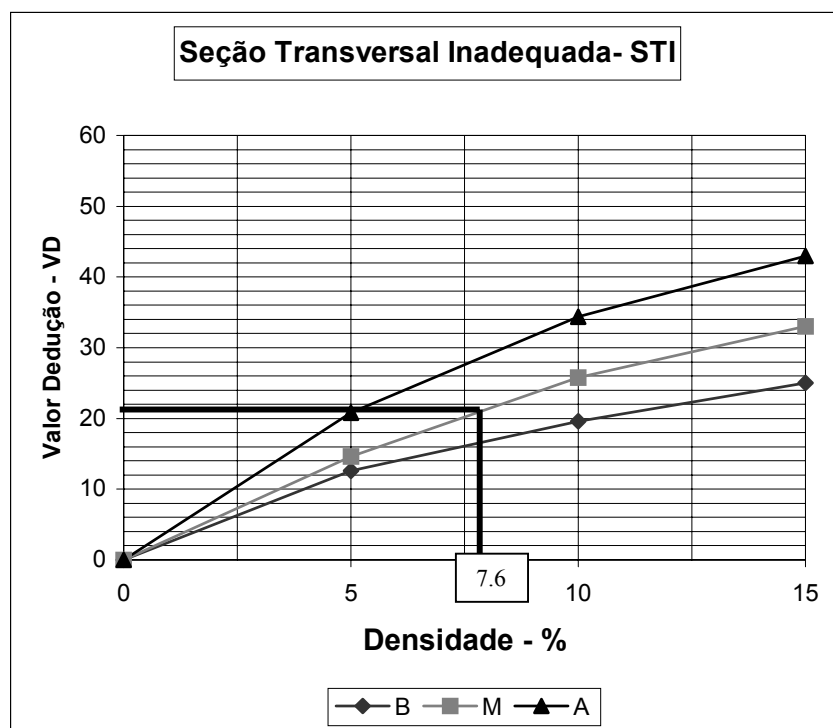
Figura E.1. Nomograma do STI – Valor-dedução para a densidade 7.6% e nível de severidade médio
