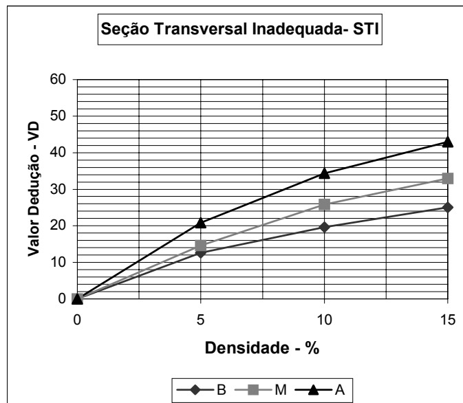
Figura B.1. Nomograma de curvas de valor-dedução – VDu: STI - Seção Transversal Inadequada
