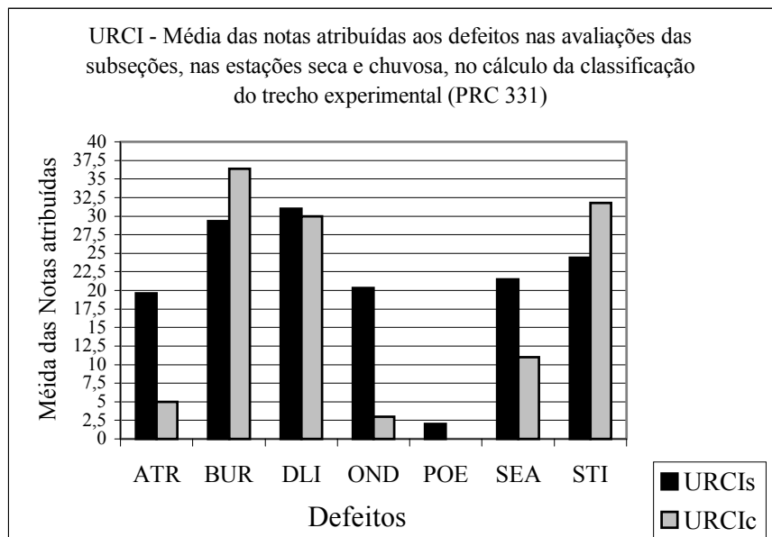
Figura 6.16. URCI - Média das notas atribuídas aos defeitos nas avaliações das subseções, nas estações seca e chuvosa, no cálculo da classificação do trecho experimental (PRC 331)
