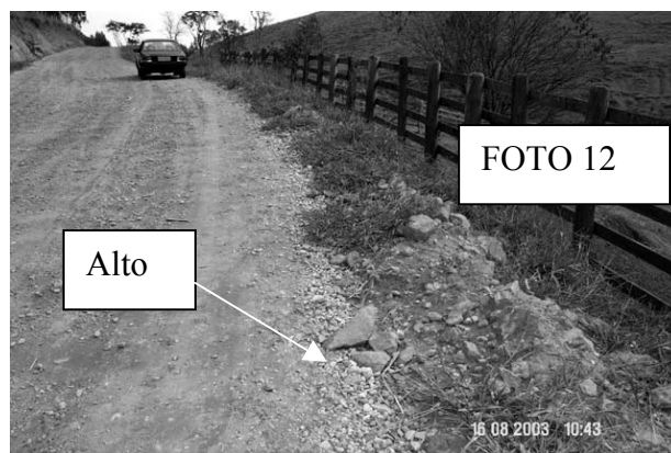
Figura 6.23. Segregação de Agregados: bermas nas laterais – fotografia do nível de severidade: foto 12
