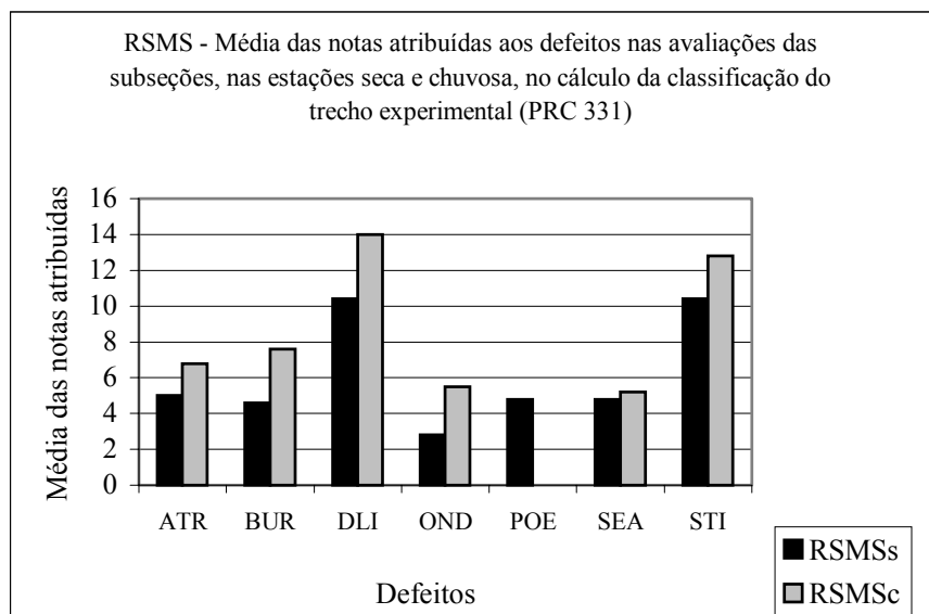
Figura 6.17. RSMS - Média das notas atribuídas aos defeitos nas avaliações das subseções, nas estações seca e chuvosa, no cálculo da classificação do trecho experimental (PRC 331)
