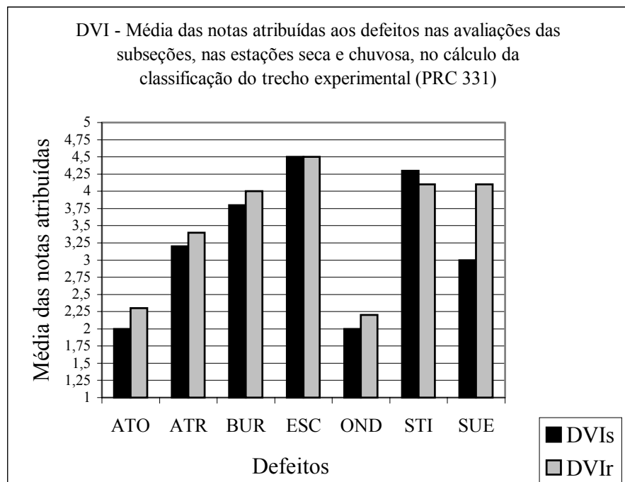
Figura 6.13. DVI e DVIr - Média das notas atribuídas aos defeitos nas avaliações das subseções, nas estações seca e chuvosa, no cálculo da classificação do trecho experimental (PRC 331)
