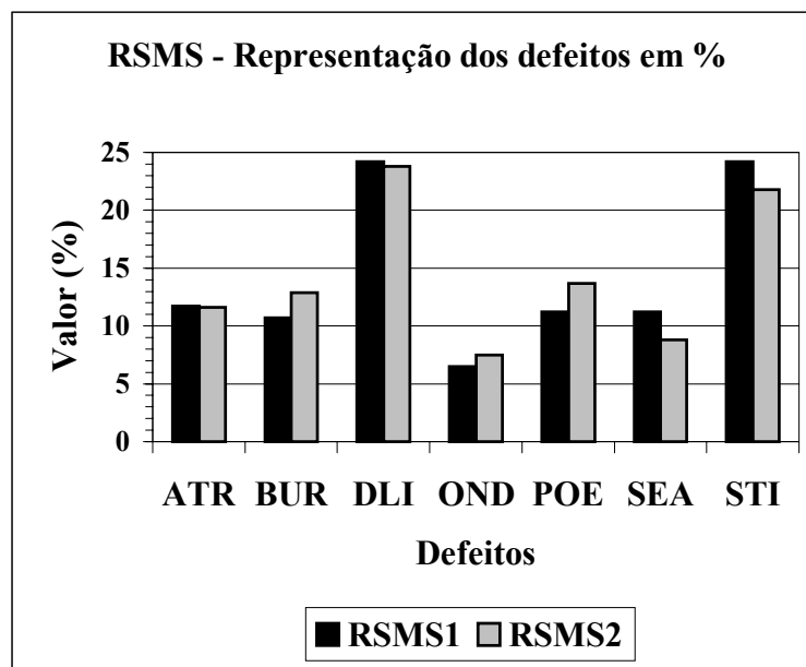
Figura 7.7. RSMS - Gráfico da representação dos defeitos em %, na avaliação da estação seca – RSMS1 e da chuvosa – RSMS2
