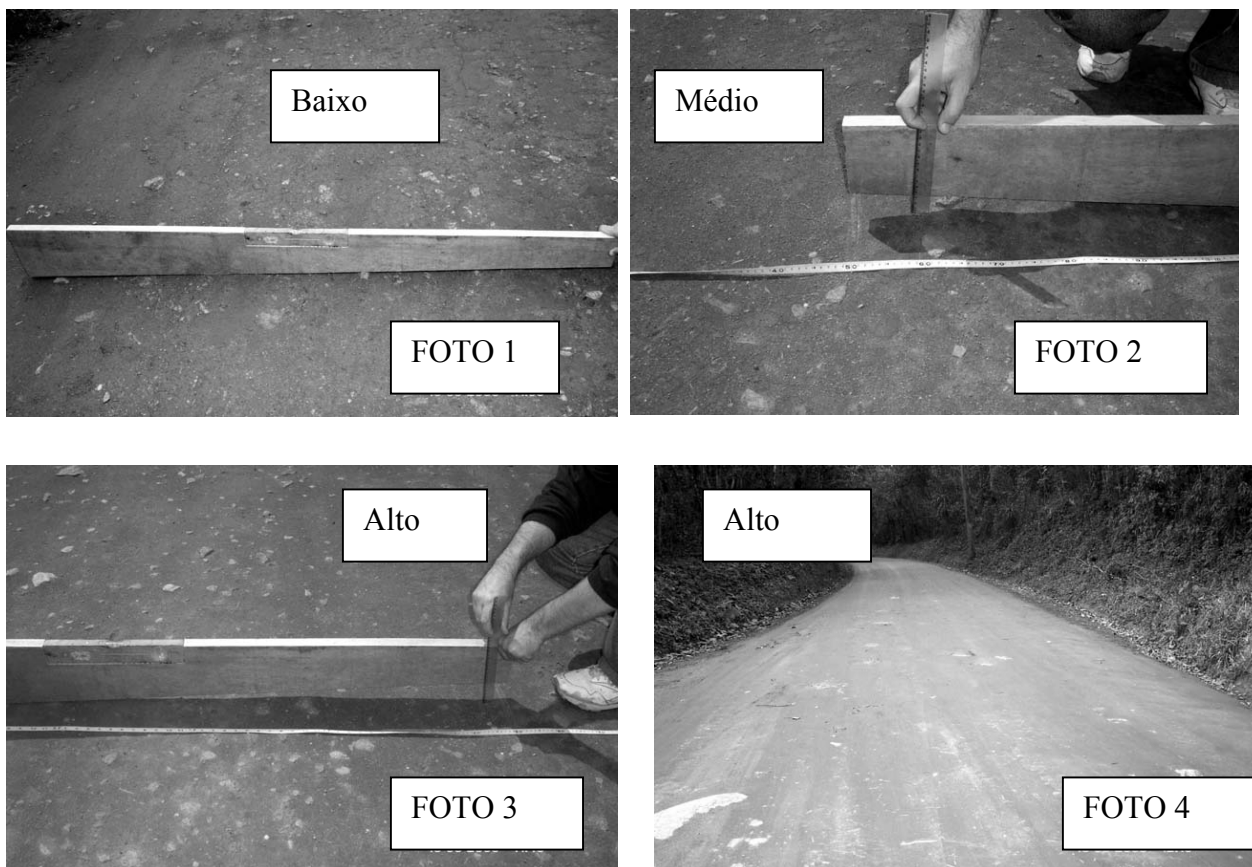
Figura 6.18. Seção transversal Inadequada – fotografias dos níveis de severidade: fotos- 1, 2, 3 e 4.
