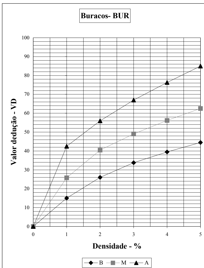
Figura B.5. Nomograma de curvas de valor-dedução – VD u : BUR - Buracos
