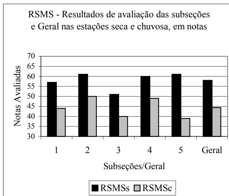
Figura 6.11. RSMS – Resultados de avaliação das subseções e geral nas estações seca e chuvosa, em notas
