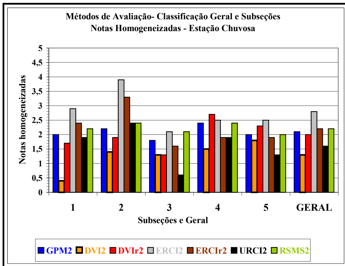
Figura 7.2. Gráfico das notas homogeneizadas das subseções e geral pelos métodos aplicados em campo, na estação chuvosa
