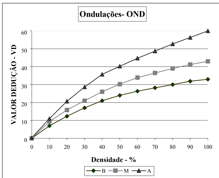
Figura B.3. Nomograma de curvas de valor-dedução – VD u : OND - Ondulações
