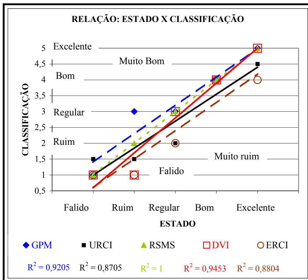
Figura 5.2. Gráfico da relação entre o estado de condição e as classificações obtidas
