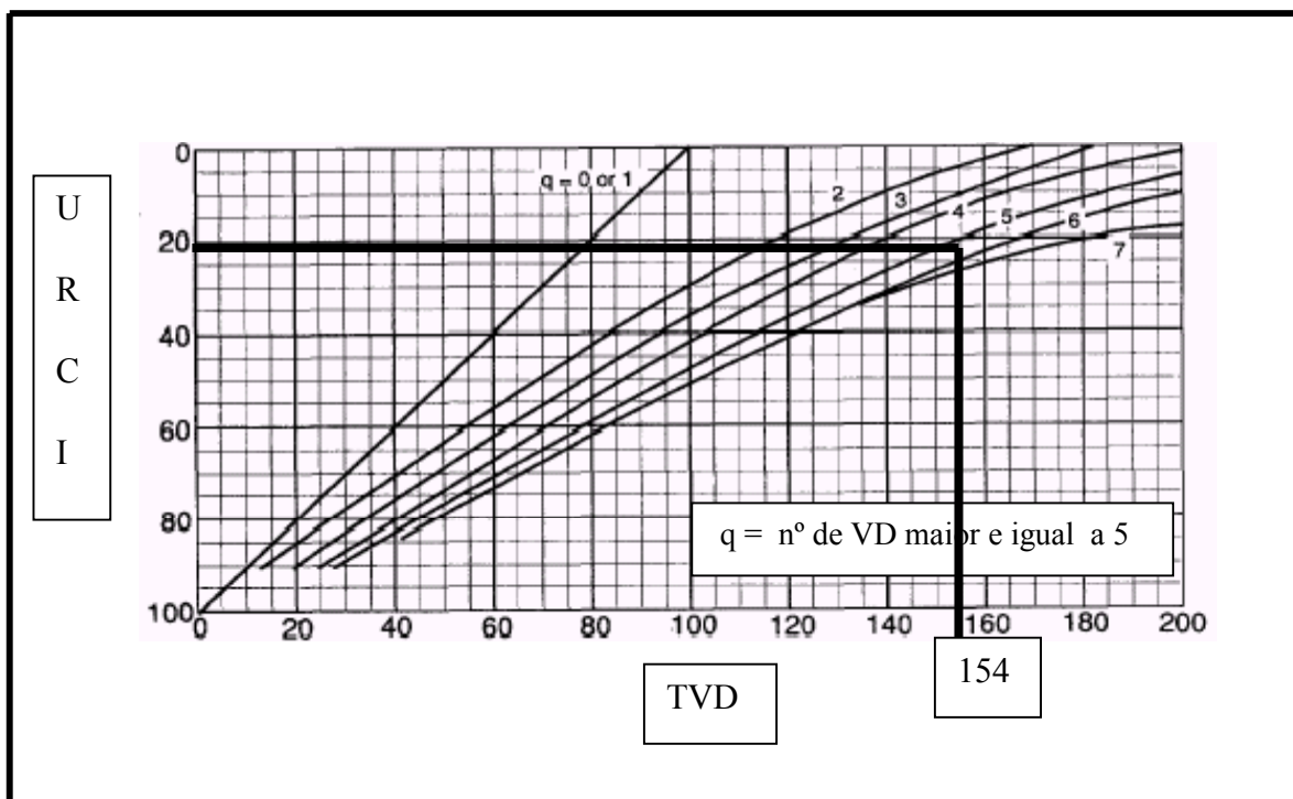
Figura E.2. Nomograma para determinação do URCI – para o TVD = 154 e q = 5 \Rightarrow \text{URCI} = 20 .
