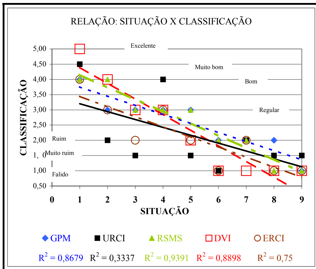
Figura 5.1. – Gráfico da relação entre a situação e classificação dos níveis de severidade e densidade dos defeitos avaliados pelos métodos de avaliação selecionados
