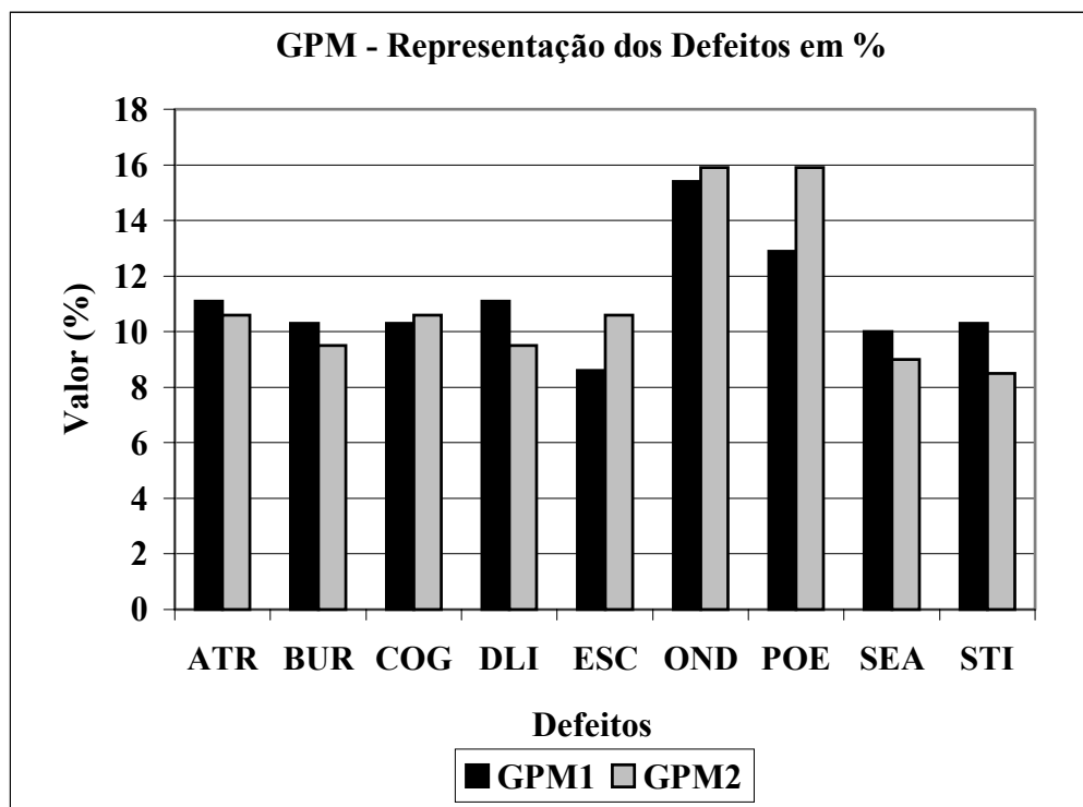
Figura 7.4. GPM - Gráfico da representação dos defeitos em %, na avaliação da estação seca – GPM1 e da chuvosa - GPM2
