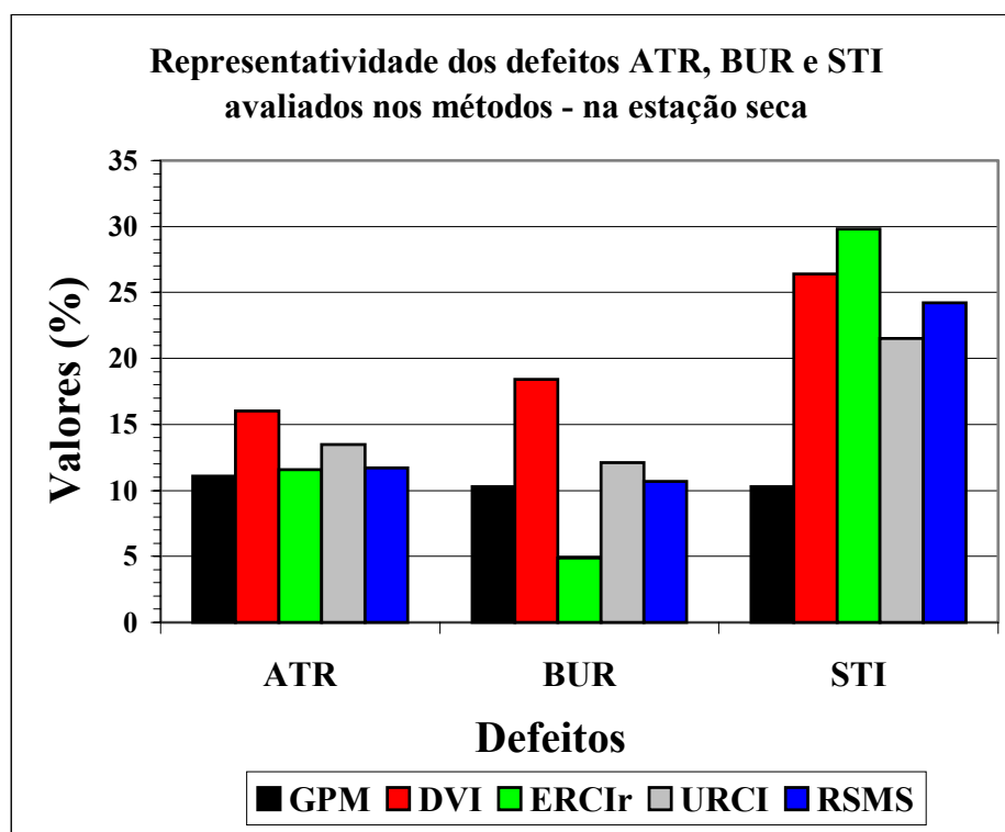
Figura 7.9. Gráfico da representatividade em % dos defeitos ATR, BUR e STI avaliados pelos métodos na estação seca
