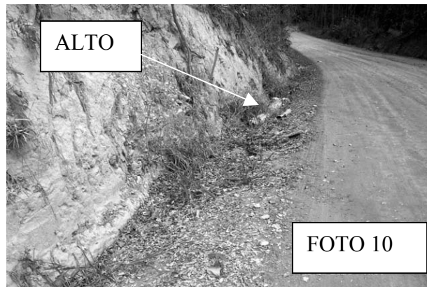
Figura 6.21. Drenagem Lateral - níveis de severidade: fotos- 8, 9 e 10
