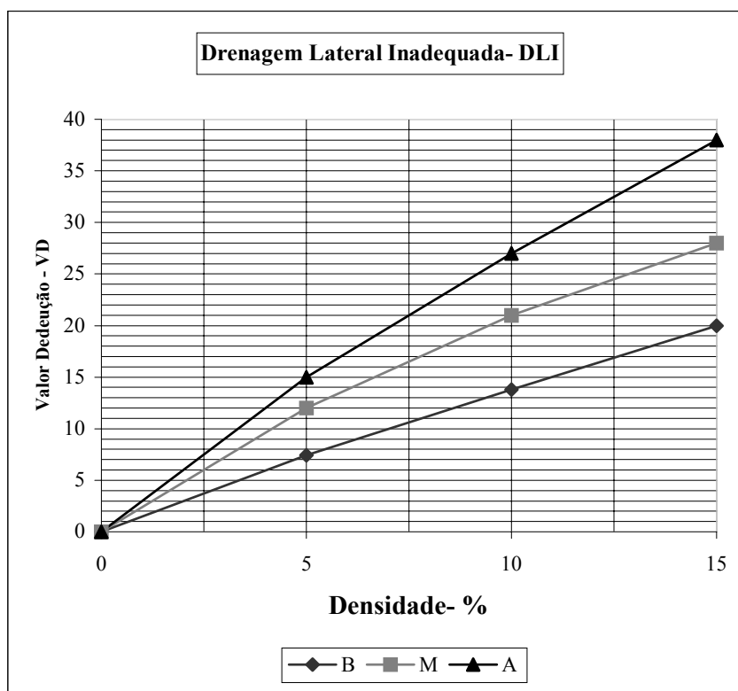
Figura B.2. Nomograma de curvas de valor-dedução – VD u : DLI - Drenagem Lateral Inadequada
