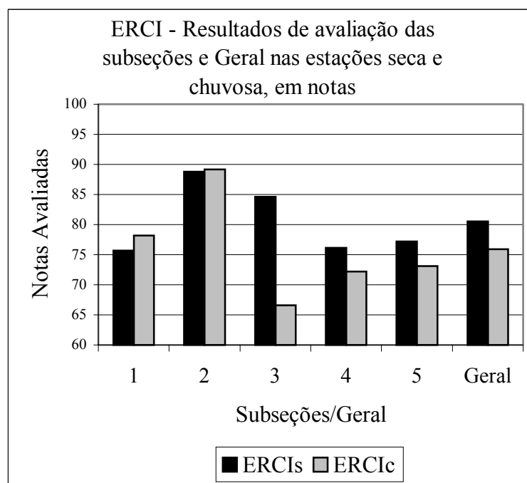
Figura 6.8. ERCI – Resultados de avaliação das subseções e geral nas estações seca e chuvosa, em notas
