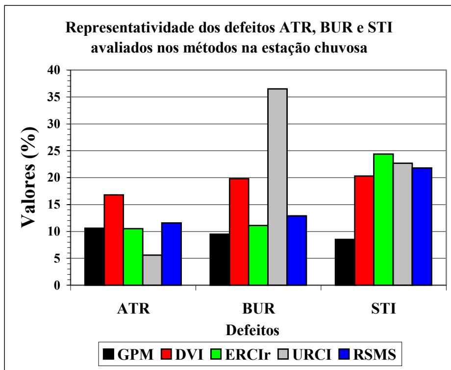
Figura 7.10. Gráfico da representatividade em % dos defeitos ATR, BUR e STI avaliados pelos métodos na estação chuvosa
