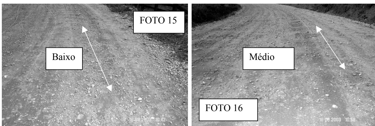
Figura 6.25. Ondulações – fotografias dos níveis de severidade: fotos 15 e 16
