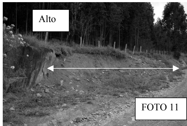
Figura 6.22. Falha no Muro de Contenção – fotografia do nível de severidade: foto 11
