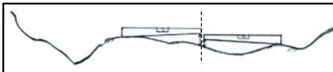
Figura 6.19. Croqui de situação de medição do defeito STI com o gabarito de bolha, diferença entre as medidas de cada lado do eixo de uma estrada com seção “encaixada”
