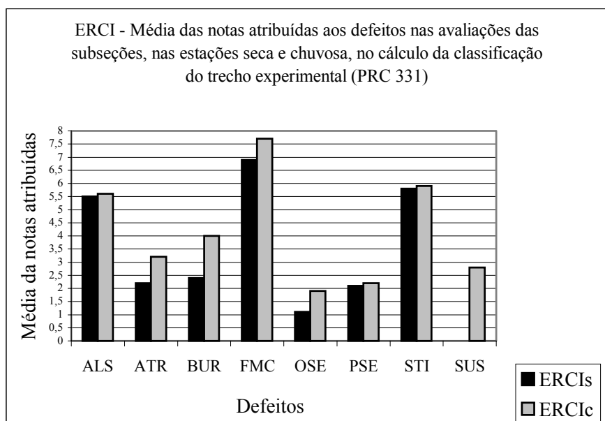
Figura 6.14. ERCI - Média das notas atribuídas aos defeitos nas avaliações das subseções, nas estações seca e chuvosa, no cálculo da classificação do trecho experimental (PRC 331)
