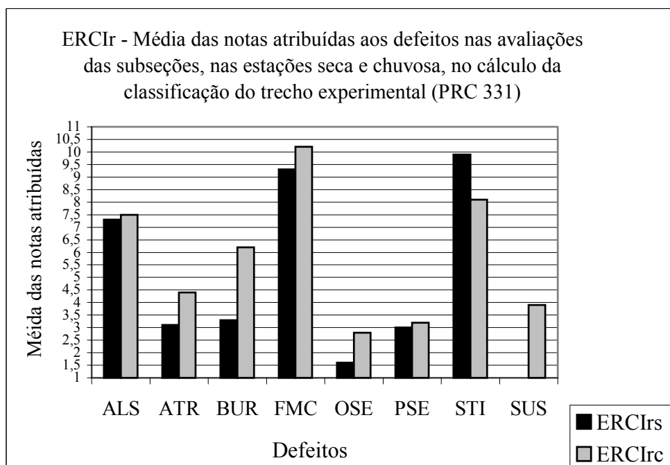
Figura 6.15. ERCIR - Média das notas atribuídas aos defeitos nas avaliações das subseções, nas estações seca e chuvosa, no cálculo da classificação do trecho experimental (PRC 331)
